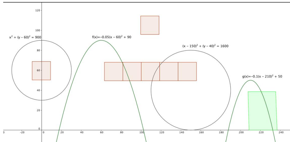
Figure 6. Modélisation mathématique des trajectoires du robot par l'équipe 3
